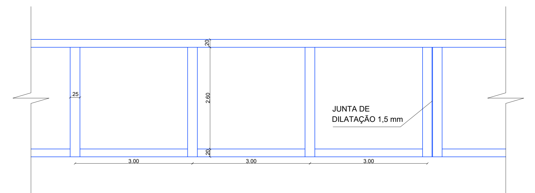
DETALHAMENTO DE MURO ESCALA 1:20
