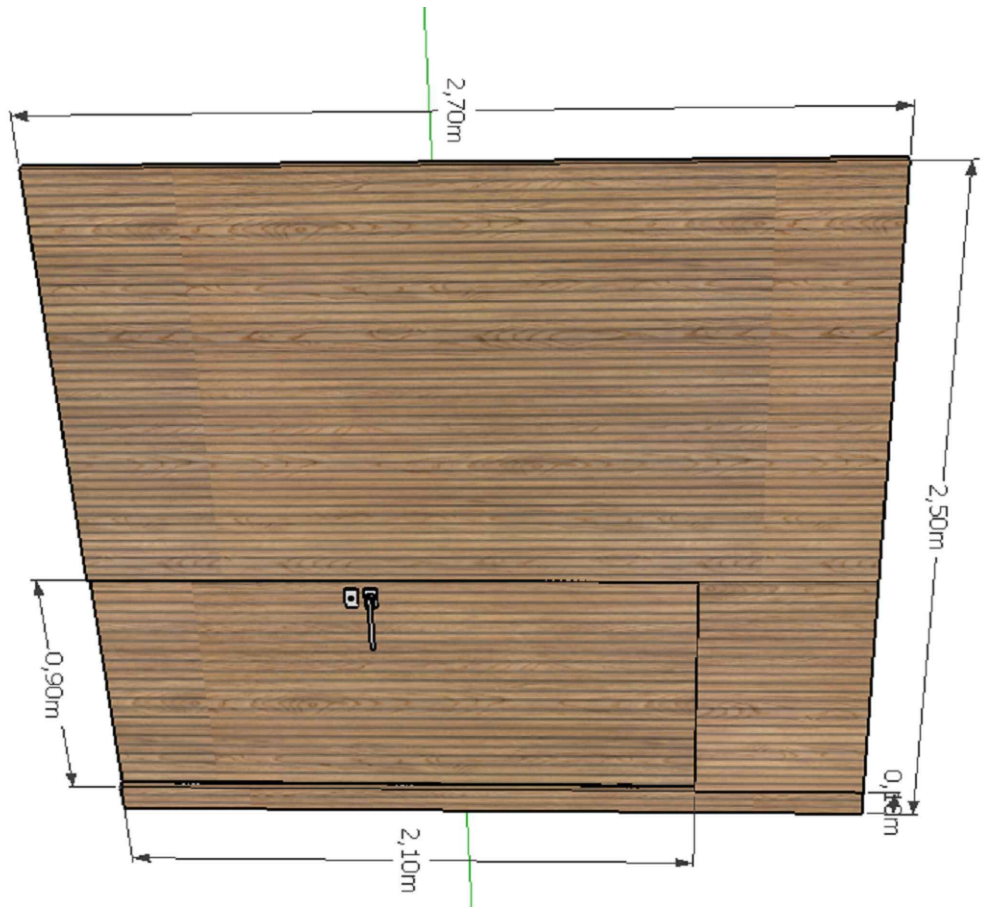
P-01 DET. PAINEL COM PORTA V-01 ESCALA 1:100
