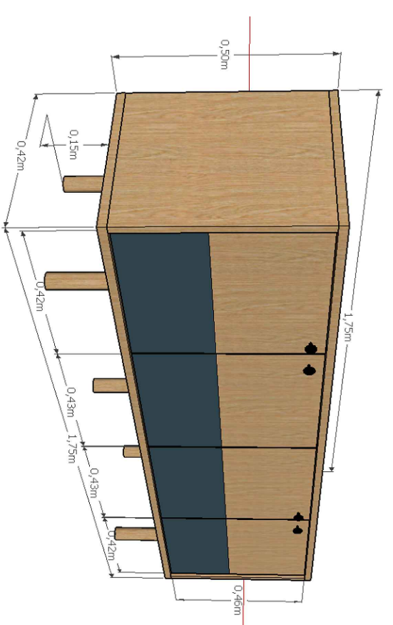
P-01 PERSPECTIVA V-01 ESCALA 1:100
