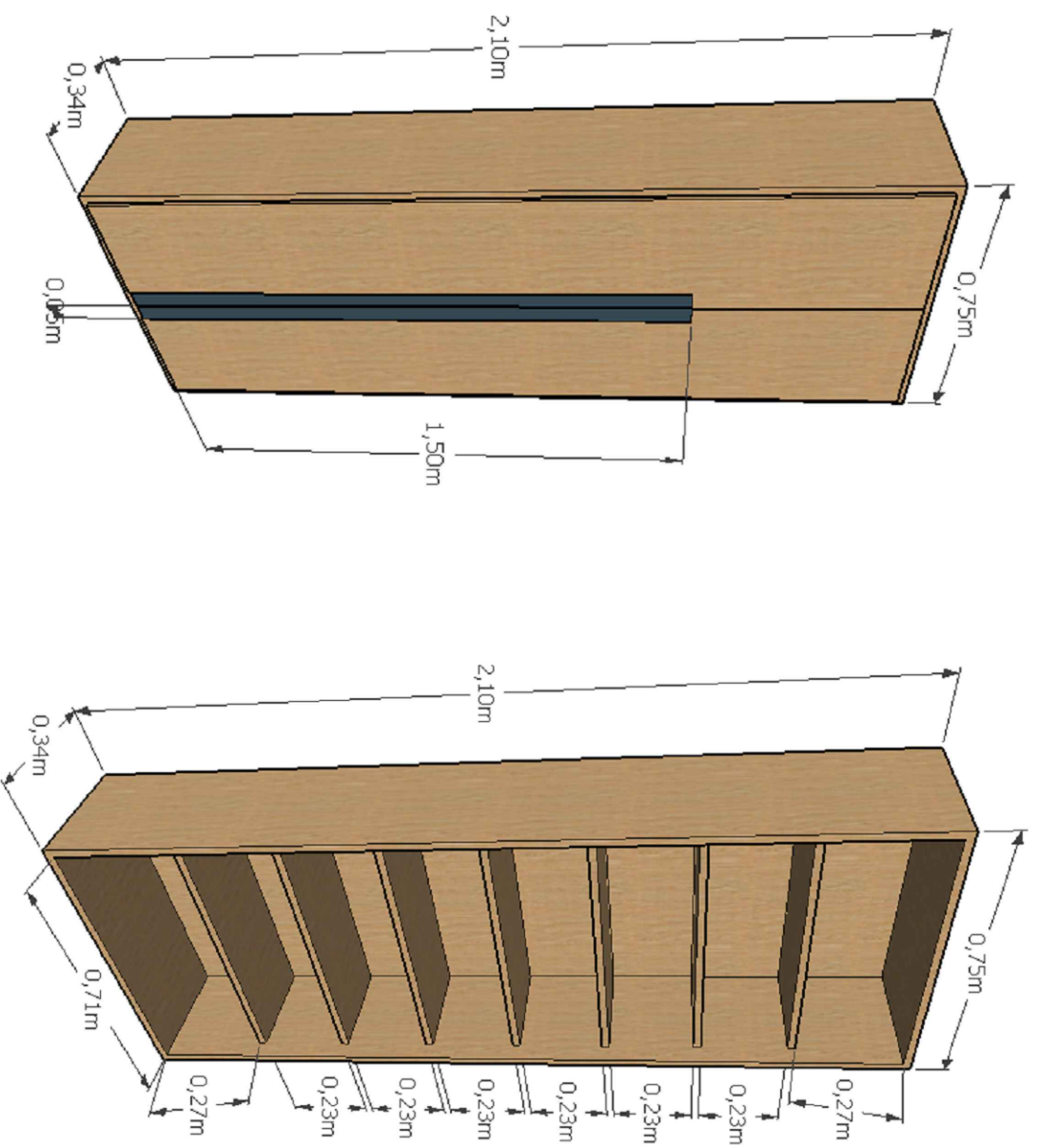
P-01 DET. ARMÁRIO V-01 ESCALA 1:100
