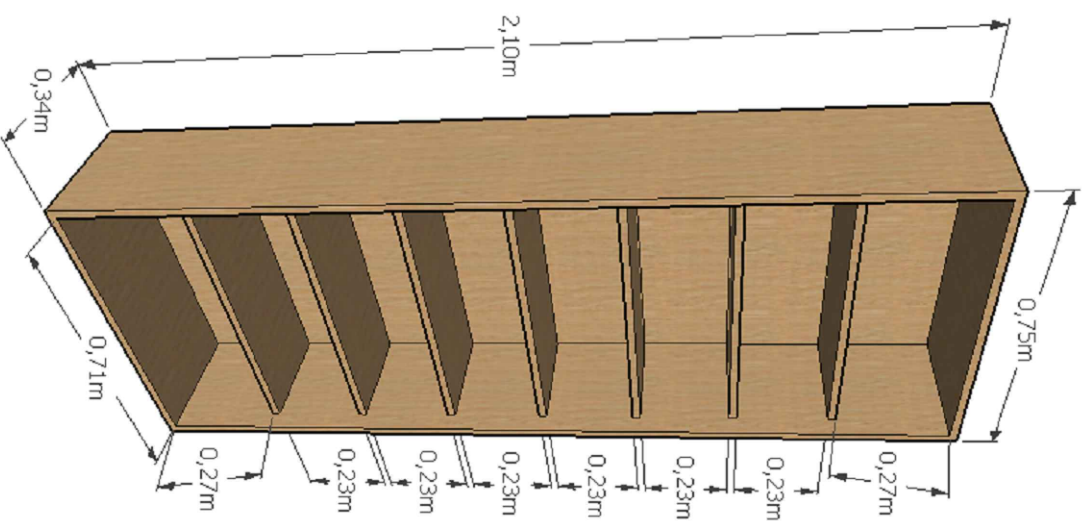
P-01 DET. ARMÁRIO - ABERTO V-01 ESCALA 1:100
