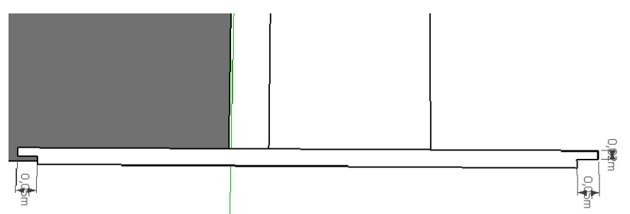
P-01 DET. RECUO PARA ILUMINAÇÃO INFERIOR E SUPERIOR DO PAINEL 1:100 ESCALA
