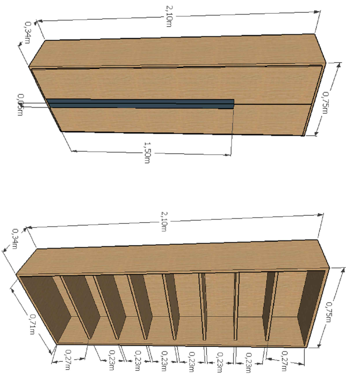
P-01 DET. ARMÁRIO V-01 ESCALA 1:100
