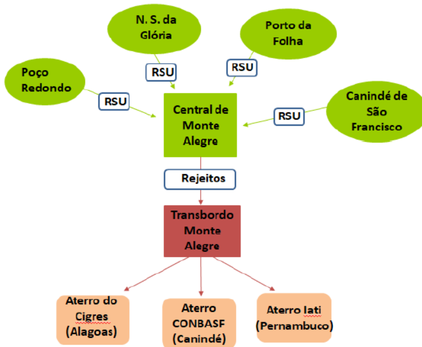
Fluxograma 03: Arranjo da Central de Triagem e Compostagem de Monte Alegre e o destino dos resíduos sólidos urbanos.
