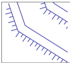
Detalhe dos taludes Declividade 1:2,5
