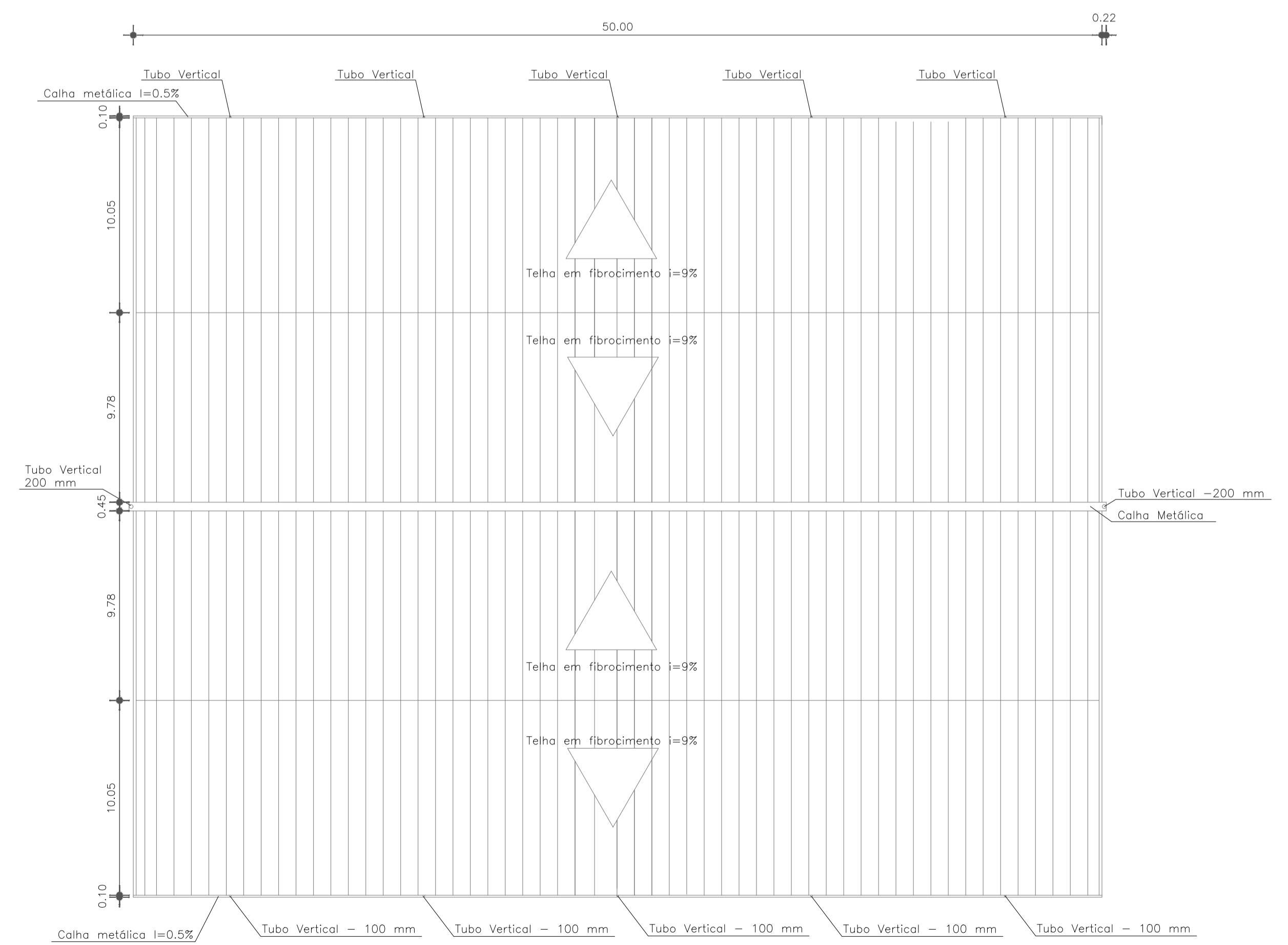
Planta de Coberta Escala 1:200
