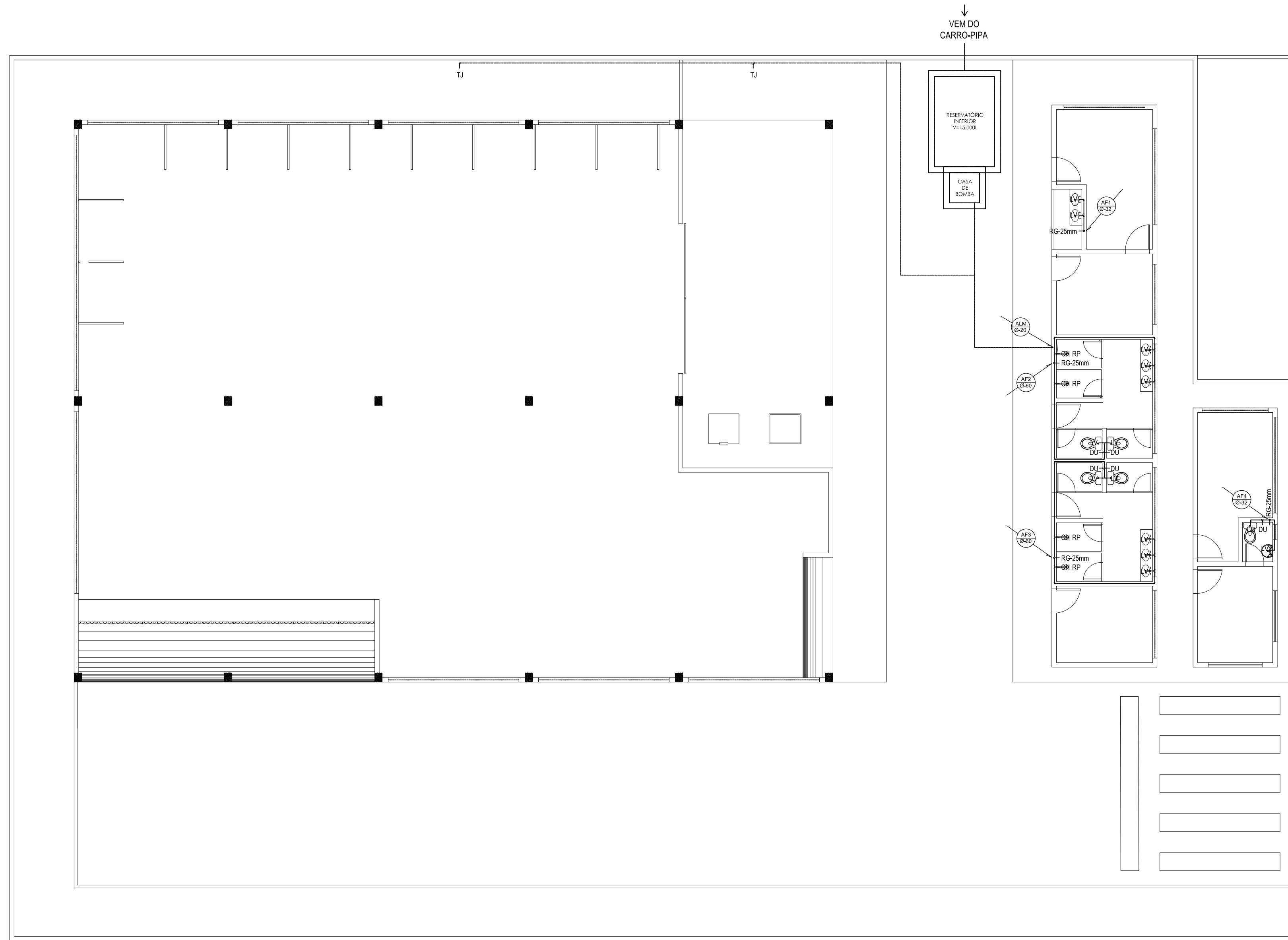
INSTALAÇÃO HIDRÁULICA PLANTA BAIXA ESCALA 1/100
