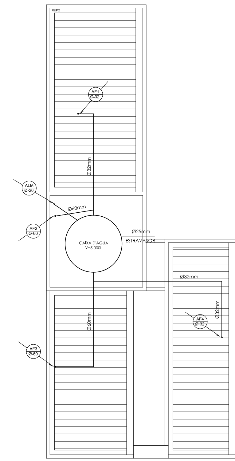
INSTALAÇÃO HIDRÁULICA COBERTURA ESCALA 1/100
