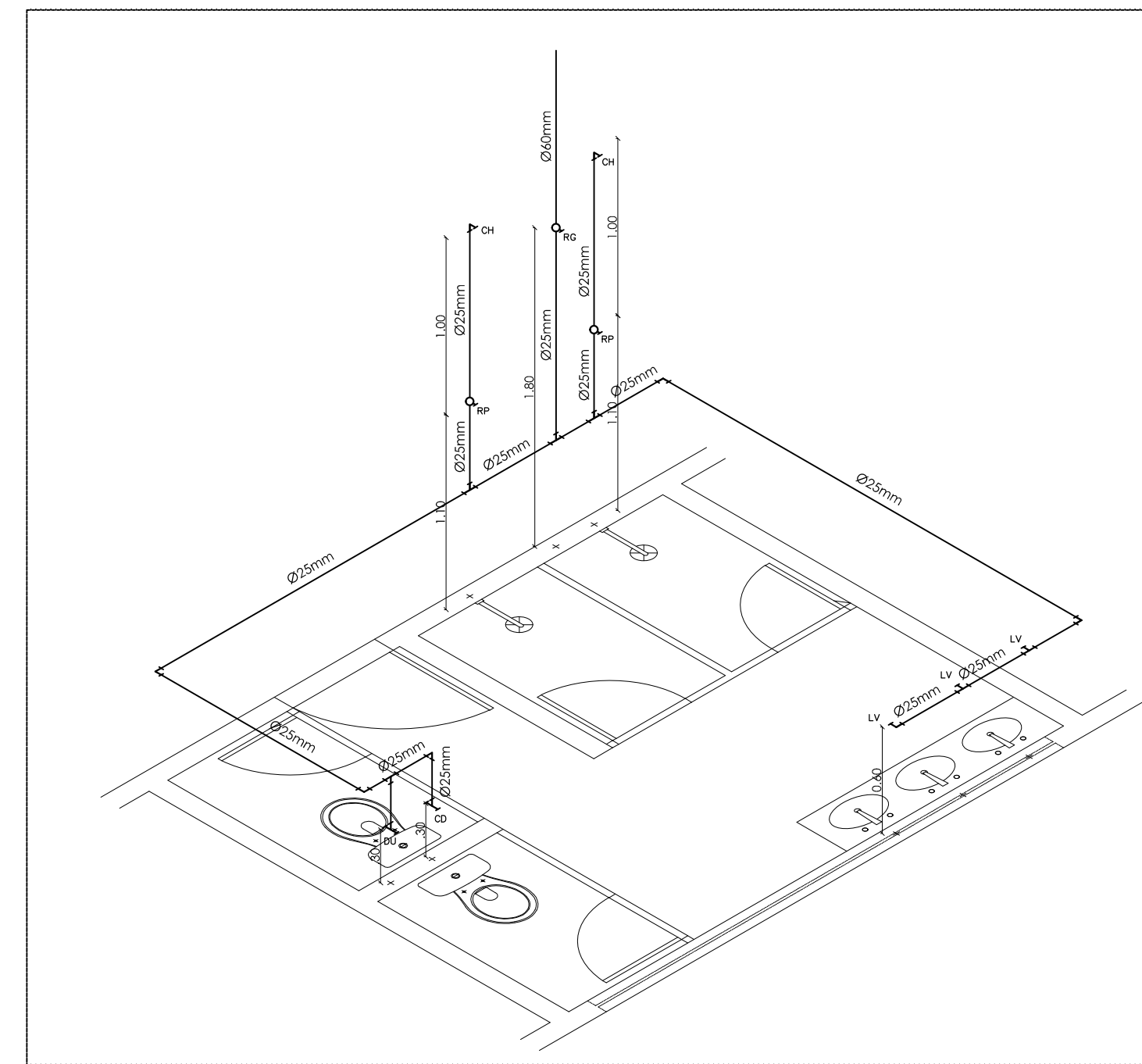
ISOMÉTRICO BWC FEM. ESCALA 1/25
