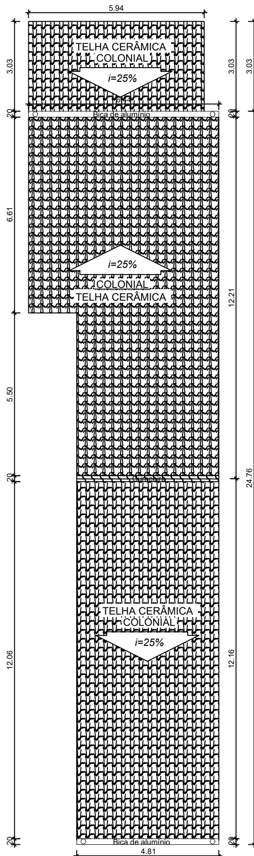
4 PLANTA DE COBERTURA ESC.: 1:125
