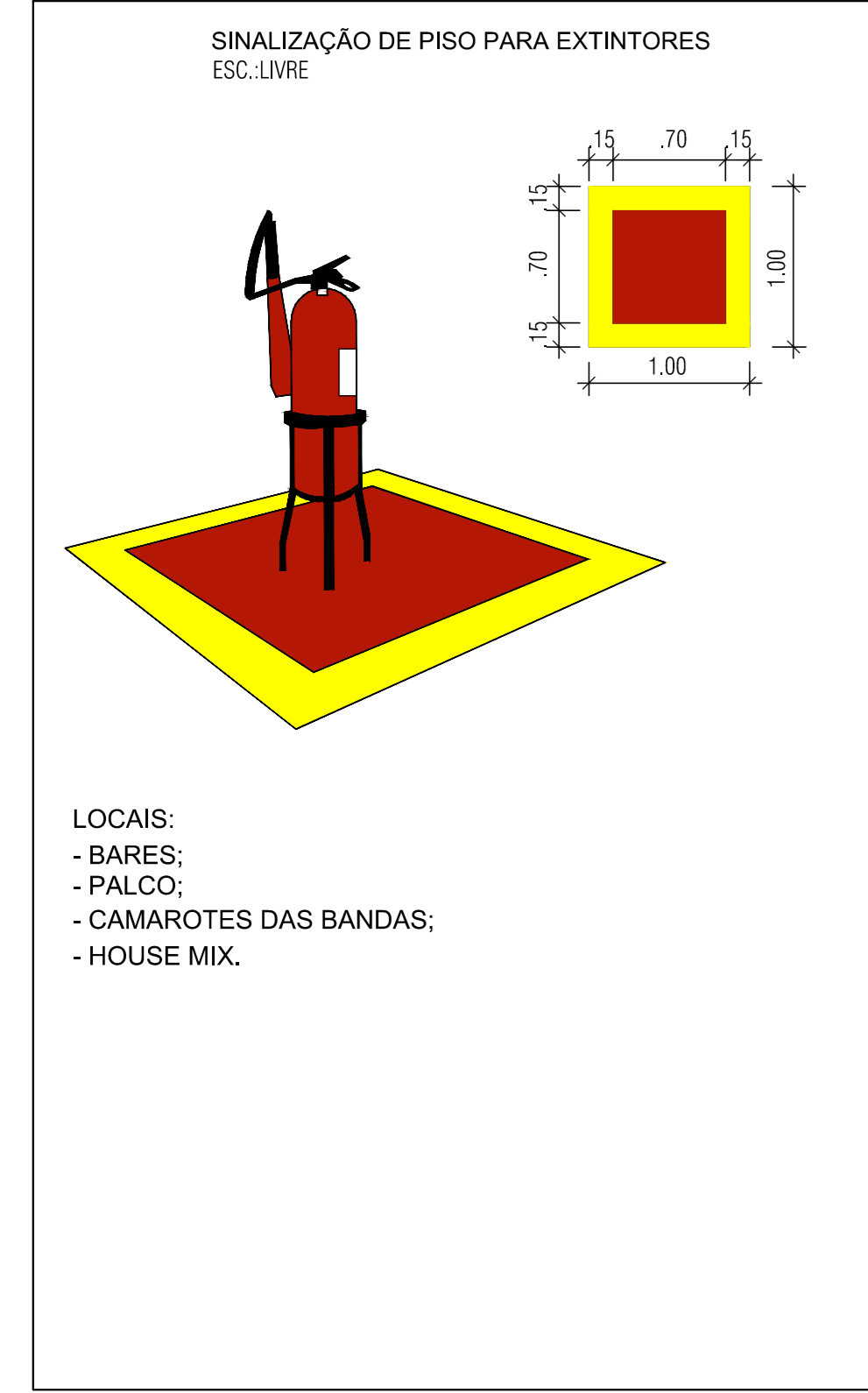
DETALHE 01 - EXTINTOR DE PISO SEM ESCALA
