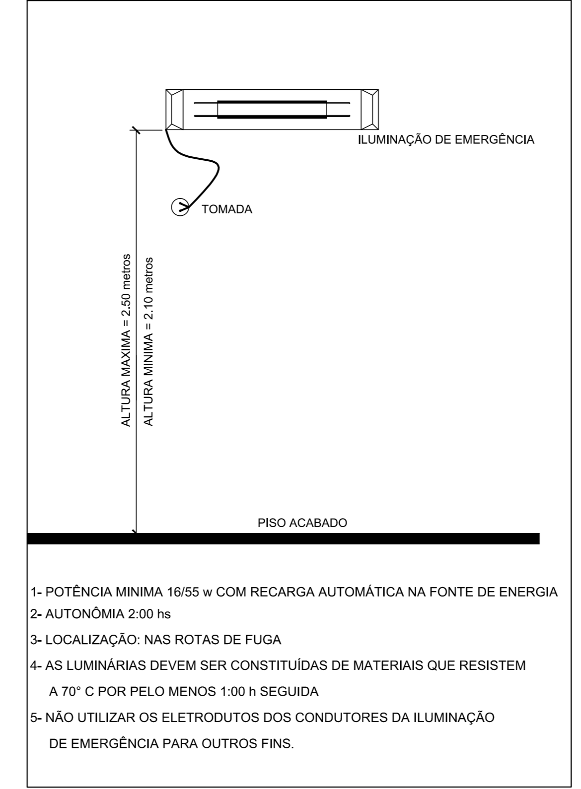
DETALHE 04 - ILUMINAÇÃO DE EMERGÊNCIA SEM ESCALA
