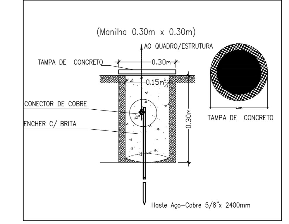
DETALHE 05 - CAIXA DE ATERRAMENTO SEM ESCALA
