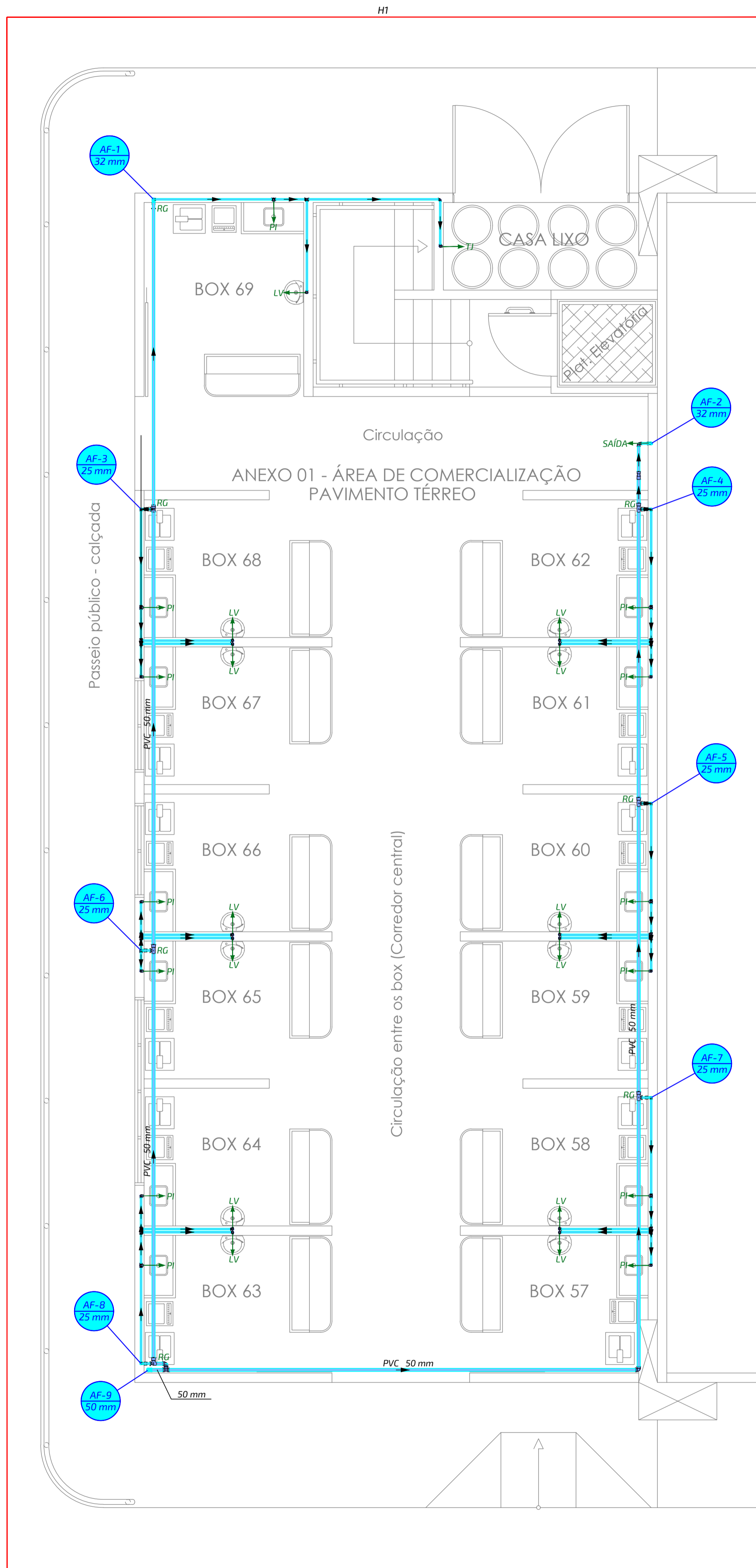
PLANTA BAIXA - PAVIMENTO TÉRREO Escala 1:50
