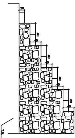
DETALHE 01 ESC. 1:50
