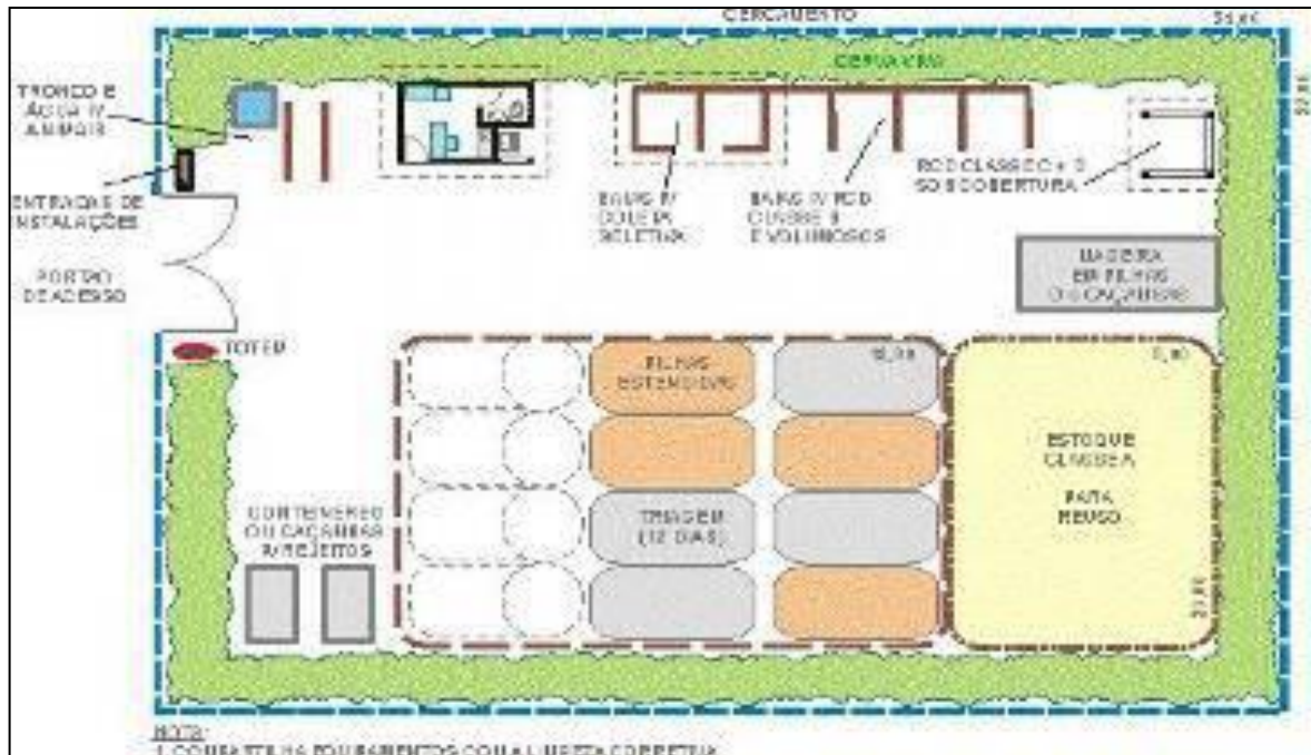
Figura 91: Layout típico para PEV Central Simplificado. Fonte: MMA (2010).
